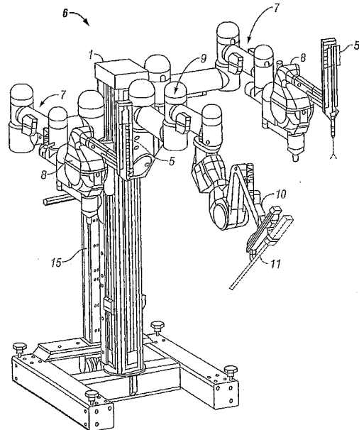
FIG. 2 (先行技術)
